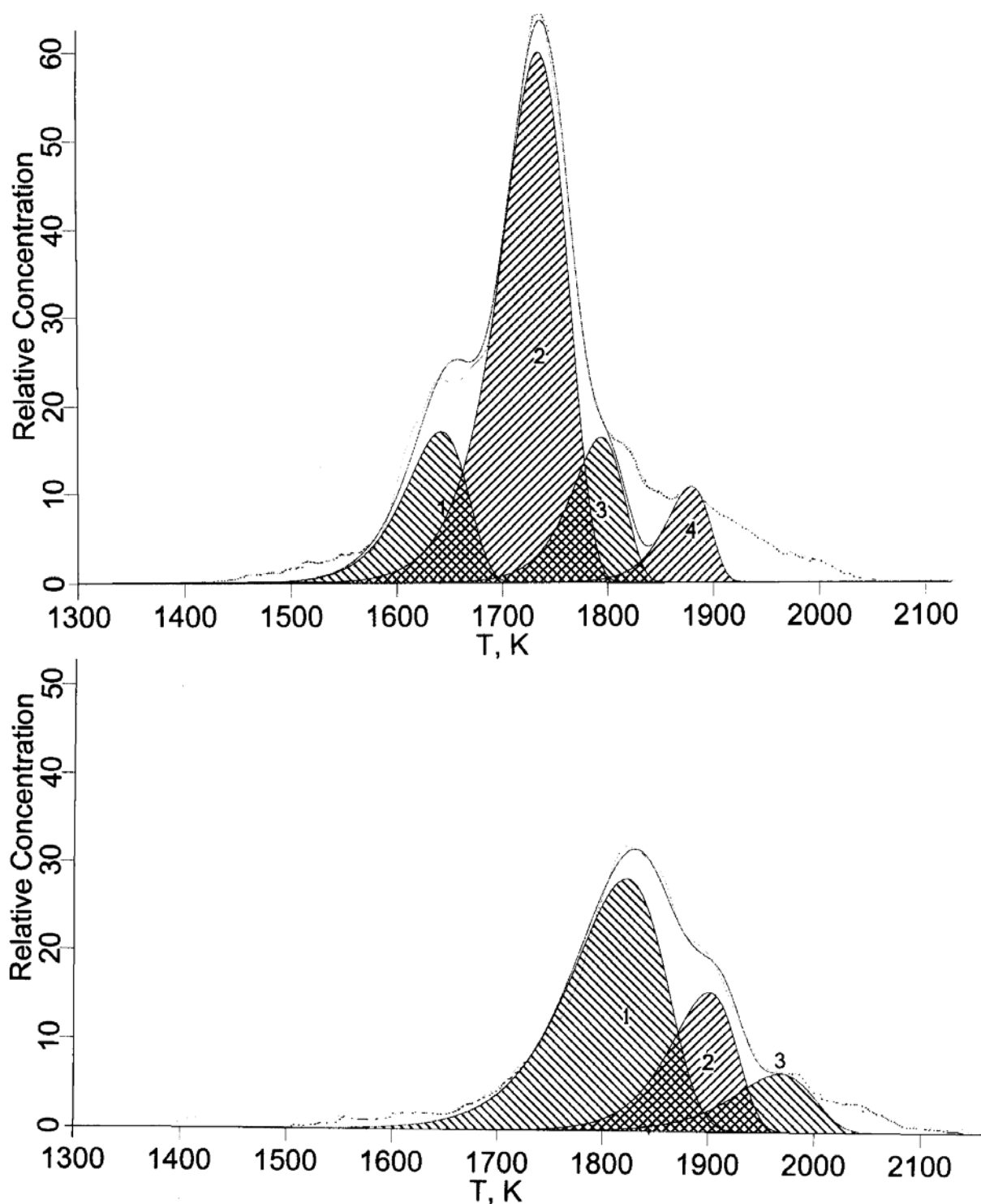
Рис 6 Кривые газовыделения из образцов кордовой стали 1 и 2 в процессе ФГА в анализаторе ТС-436 LECO (результат обработки данных программой OxSeP).
