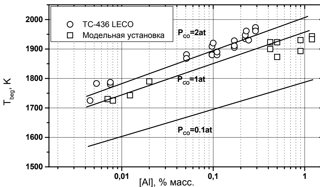
Рис. 3 Результаты исследования температур восстановления в модельной системе Fe-Al-O в зависимости от концентрации алюминия в металле и парциального давления окиси углерода P_{CO} в анализаторе. — -Расчет по приведенной модели, \bigcirc , \square - эксперимент.
