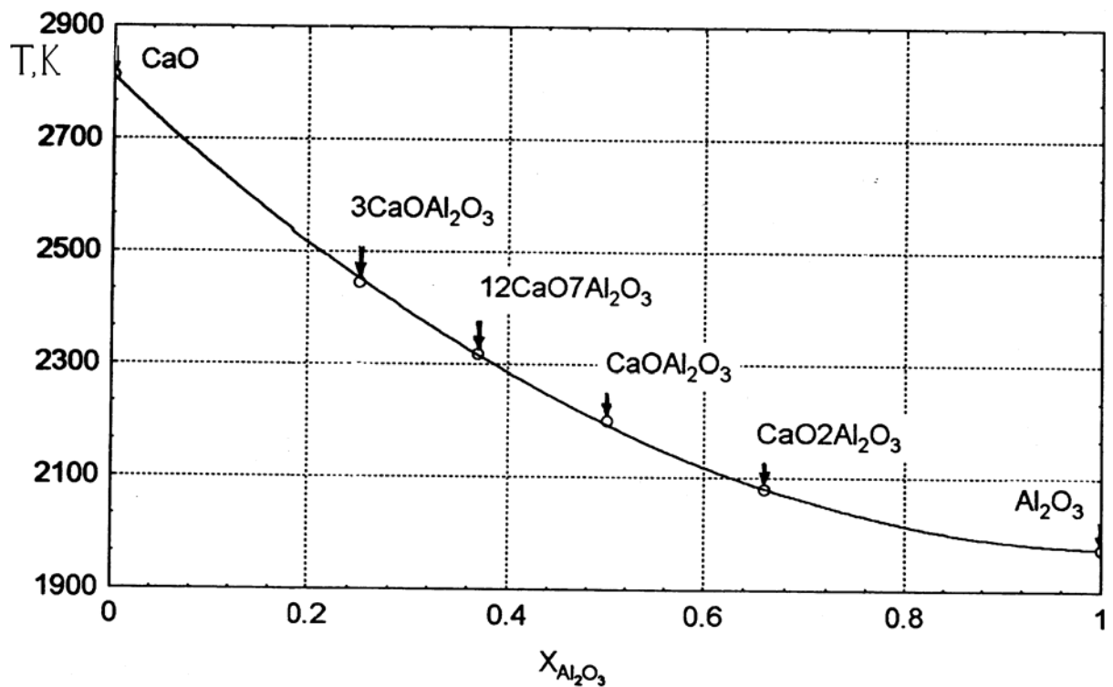
Рис. 5 Зависимость термодинамической температуры начала восстановления ( T_{beg} ) включения алюминатов кальция от активности оксида алюминия ( a_{Al_2O_3} ) в оксидной системе CaO - Al_2O_3 . (расчет).
