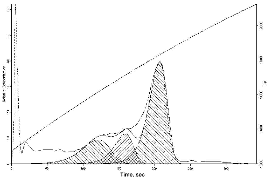
Рис 1 Кривая газовыделения из образца стали 45 раскисненной алюминием в процессе ФГА в анализаторе TC-436 LECO (результат обработки данных программой OxSeP).
